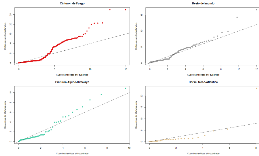
Figura 3. QQ-plots multivariantes de Mahalanobis por zona sísmica.
